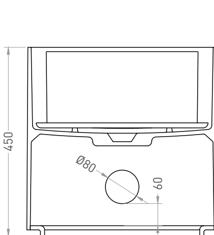
ВИД В*
